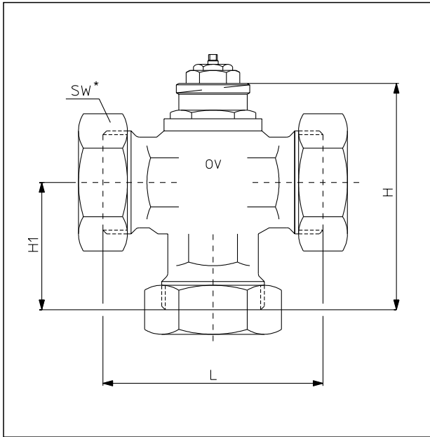
Robinetts mitigeurs et inverseurs Oventrop
