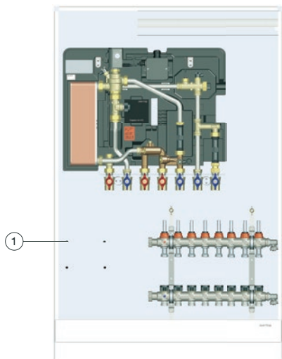
Fig. 3: Perçages préfabriqués
