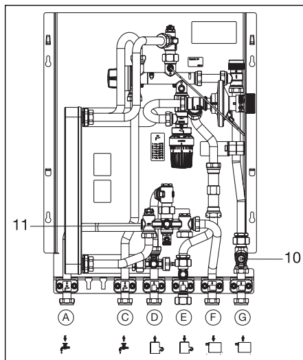
Afb. 7.1 Inbouwpositie vuulfilter
