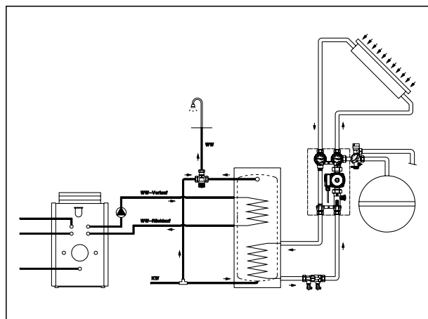
Instalacja solarna
