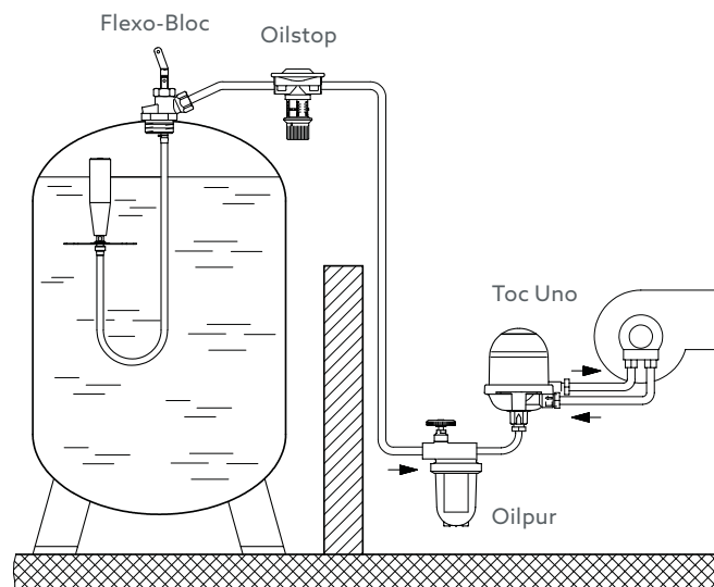
Schéma d'installation
