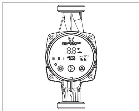
Grundfos ALPHA 2.1
