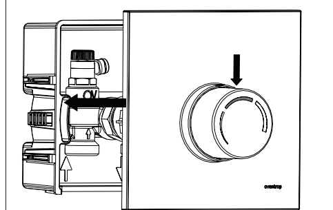
Fig. 6: Montage du capot avec poignée manuelle
