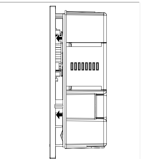
Abb. 11: Abdeckung herausgeschoben
