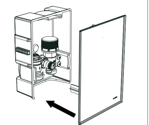
Abb. 10: Abdeckung aufsetzen
