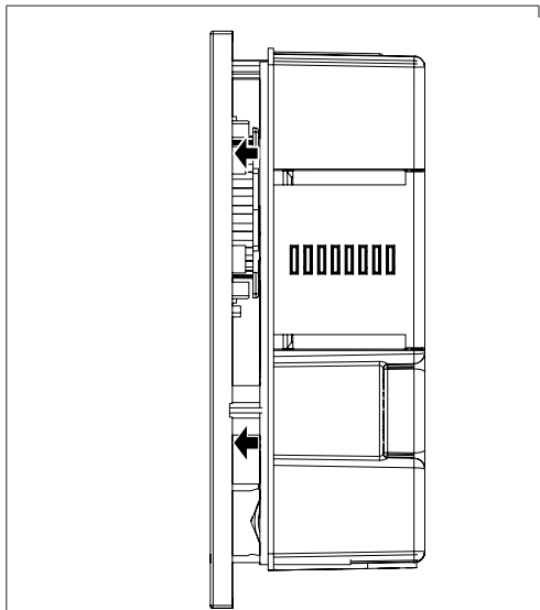
Fig. 11: Capot extrait
