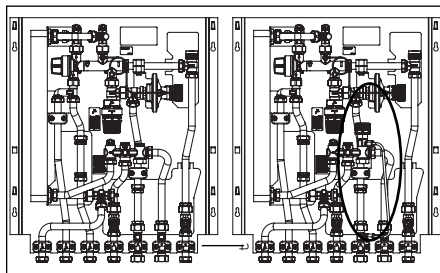
Fig. 5.1 Station d'appartement «Regudis W- HTF» avant et après le montage du set de bypass thermostatisé à consigne de température réglable
