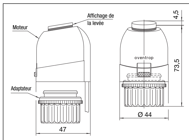
Moteurs avec fixation à griffes
