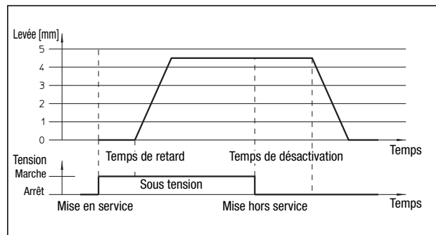
Courbe de fonctionnement – fermé hors courant
