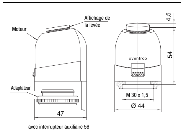
Moteurs avec raccordement fileté M 30 x 1,5
