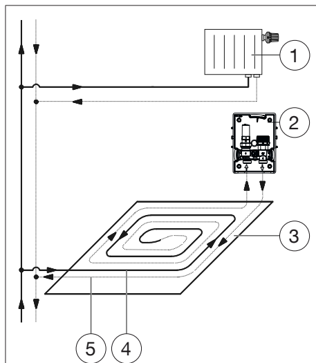
Abb. 7: Anschluss
