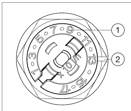
Abb. 5: Einstellung Ventileinsatz „QM“
