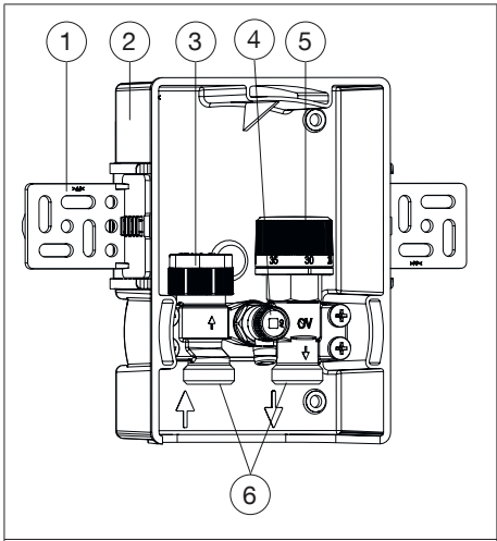
Fig. 2: Configuration de l'« Unibox TQ RTL vario »
