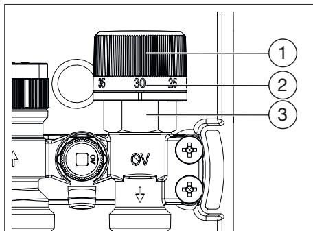
Abb. 4: Handrad
