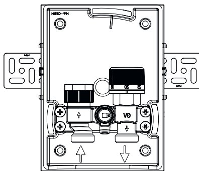
Abb. 8: „Unibox TQ RTL vario“ mit Winkeln
