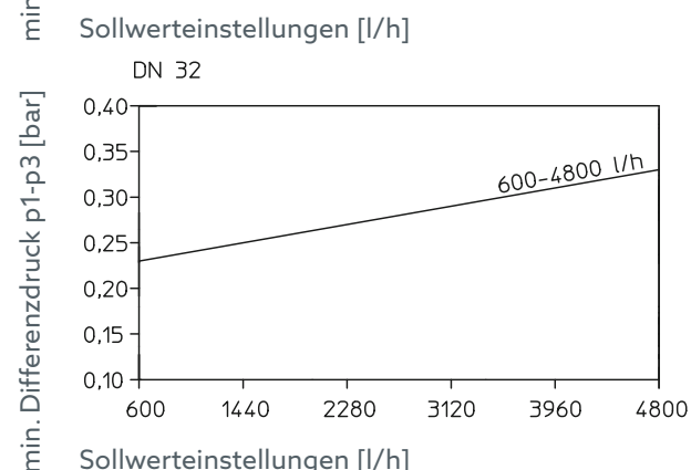
Abb. 13: Mindest-Differenzdrücke
