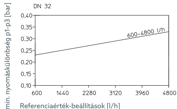
13. Minimum nyomáskülönbség
