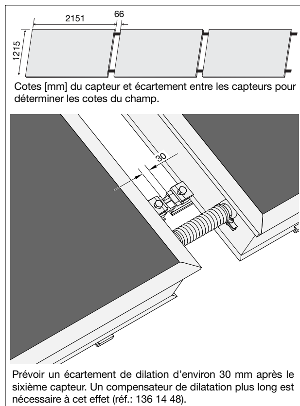
Fig. 8: Ecartements entre les capteurs
