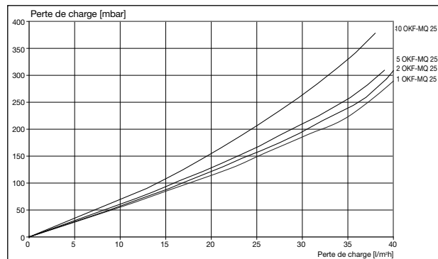
Fig. 7: Perte de charge pour plusieurs capteurs interconnectés en fonction du débit; fluide caloporteur: 40% glycol / 60% eau à 40°C; perte de charge incluant tuyaux de raccordement
