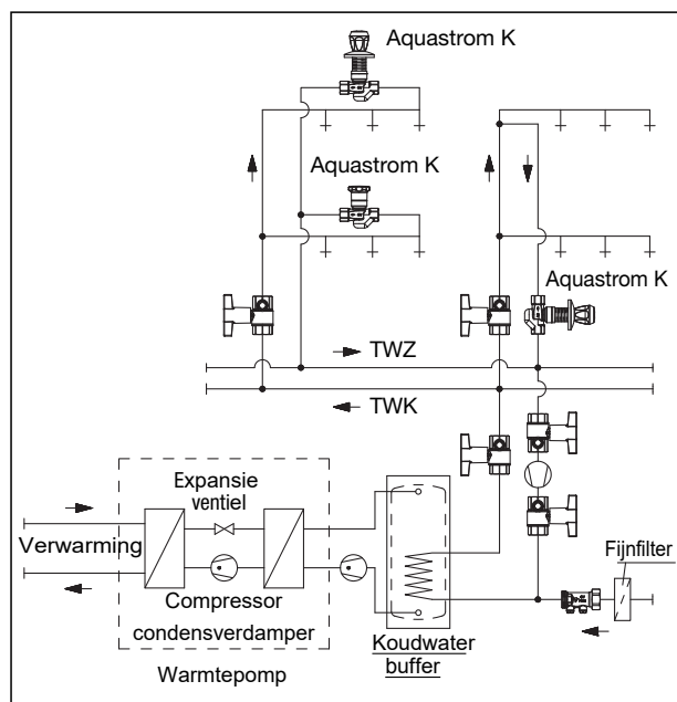
Systeemweergave warmtepomp met koudeaccumulator
