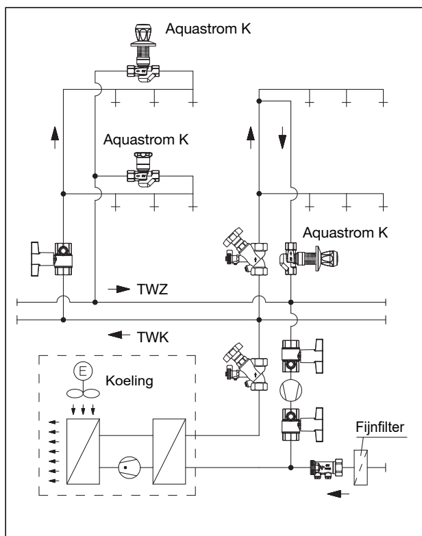
Systeemweergave met koelsysteem
