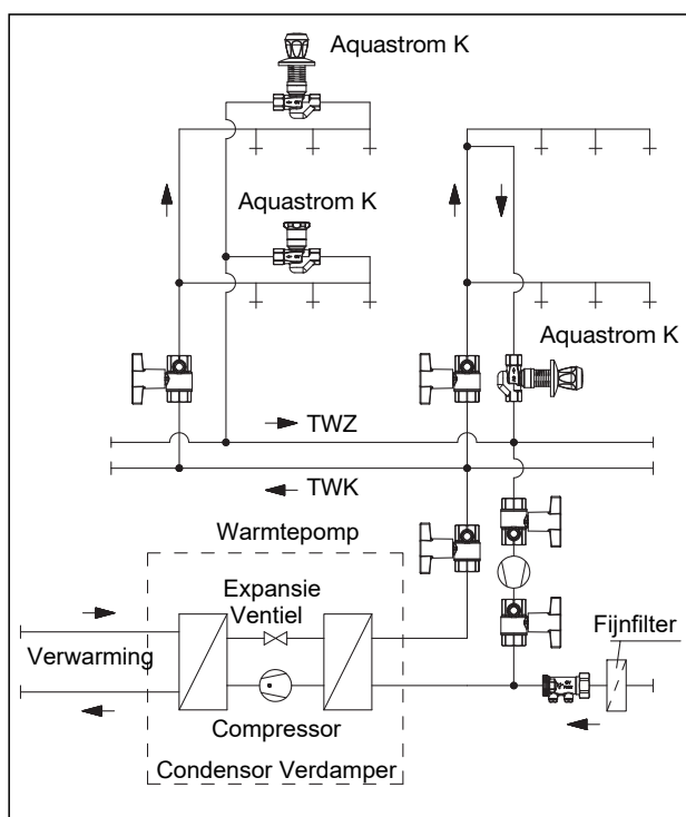
Systeemweergave met warmtepomp
