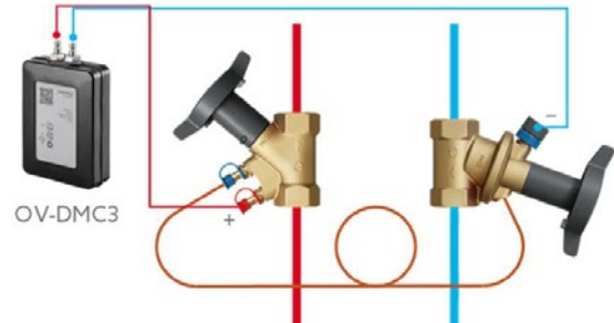
Abb. 7: Anschlussschema OV-DMC3
