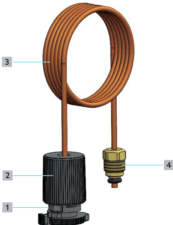
Fig. 4 - Struttura linea ad impulsi
