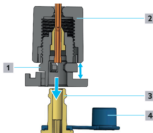
Afb. 6: Aansluiting pulsleiding op partnerventiel
