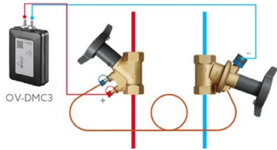
Afb. 7: Aansluitschema OV-DMC3
