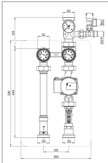
Fig. 3.1 Stazione solare "Regusol SH-180" DN32
