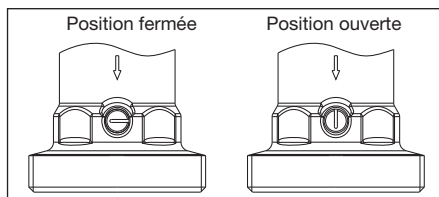
Fig. 6.1 Clapet ATS
