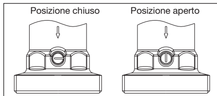
Fig. 6.1 Freno a gravità
