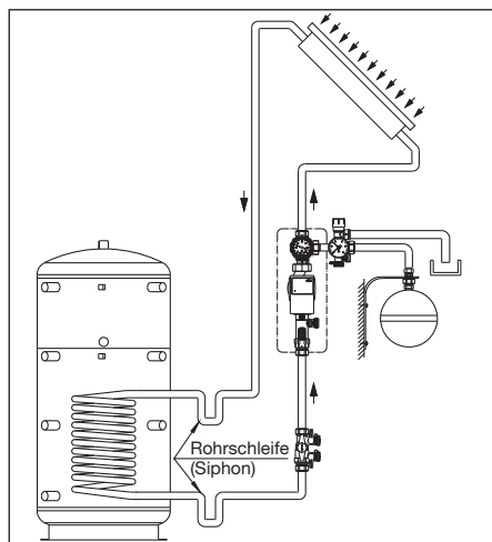
Abb. 6.2 Systembild
