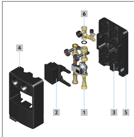
Fig. 6.6 Vue éclatée
