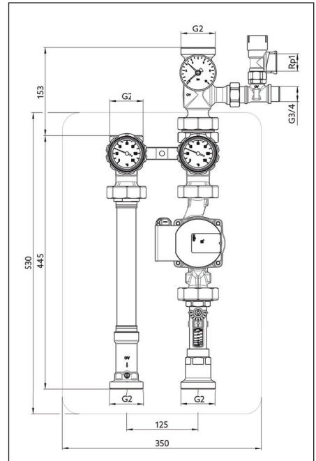
Abb. 4.1 Solarstation „Regusol SH-180“ DN32
