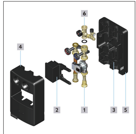
Abb. 6.6 Explosionsansicht
