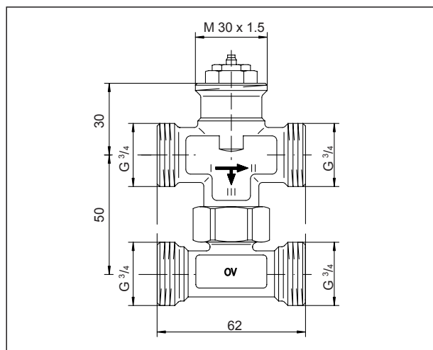
„Tri-D-plus“
