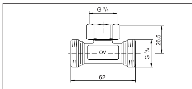
Тройник
