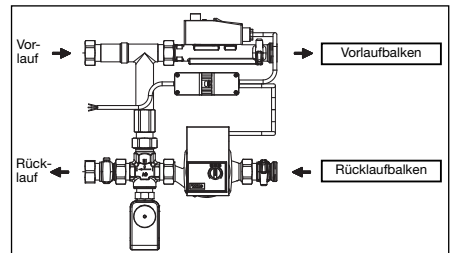
Abb. 6.2 Durchflussrichtung
