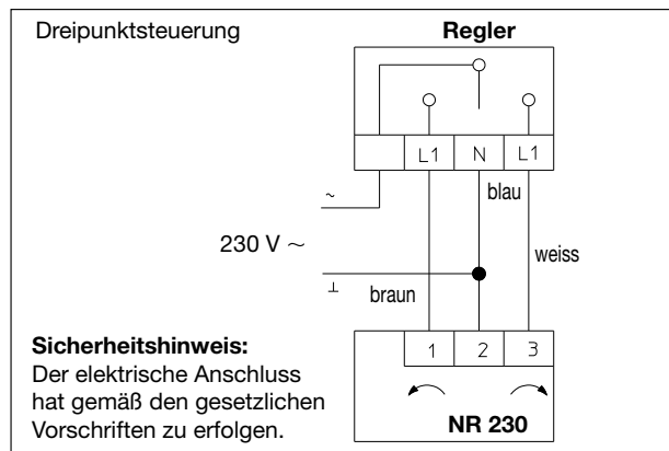
Anschluss-Schema
