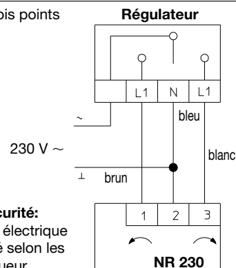
Schéma de branchement
