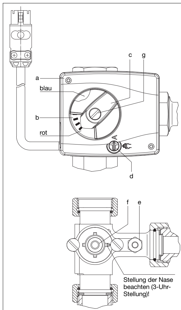
Montage Stellmotor
