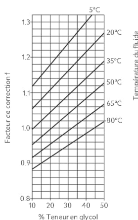
Facteur de correction f pour l'éthylène glycol
