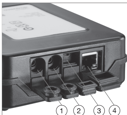
Fig. 4: Aansluitingen
