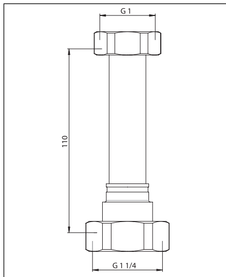
Anschlussverrohrung
