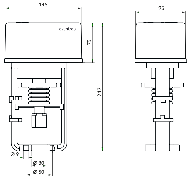
Fig. 4: Dimensions
