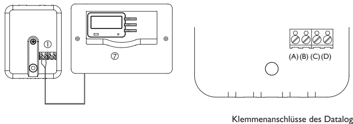
Klemmenanschlüsse des Datalog
