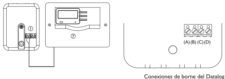
Conexiones de borne del Datalog
