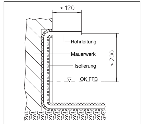
Abb. 6 Schnitt, Heizkreisanschluss
