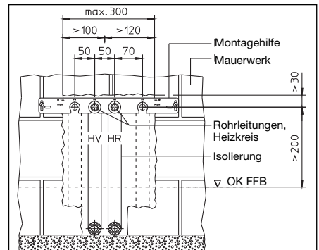
Abb. 7 Wandansicht, Heizkreisanschluss
