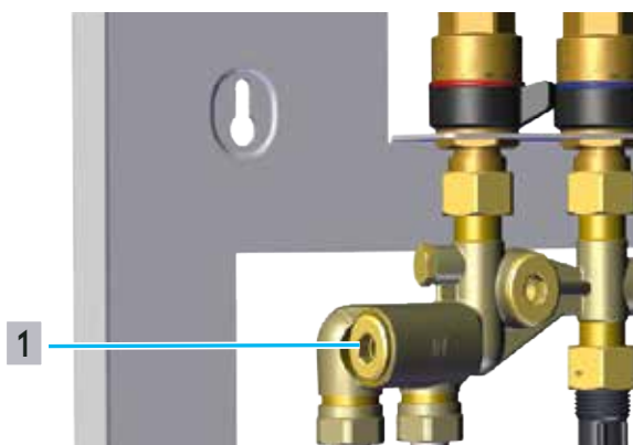
Abb. 27: Position Filtereinsatz Heizungs-Vorlauf
