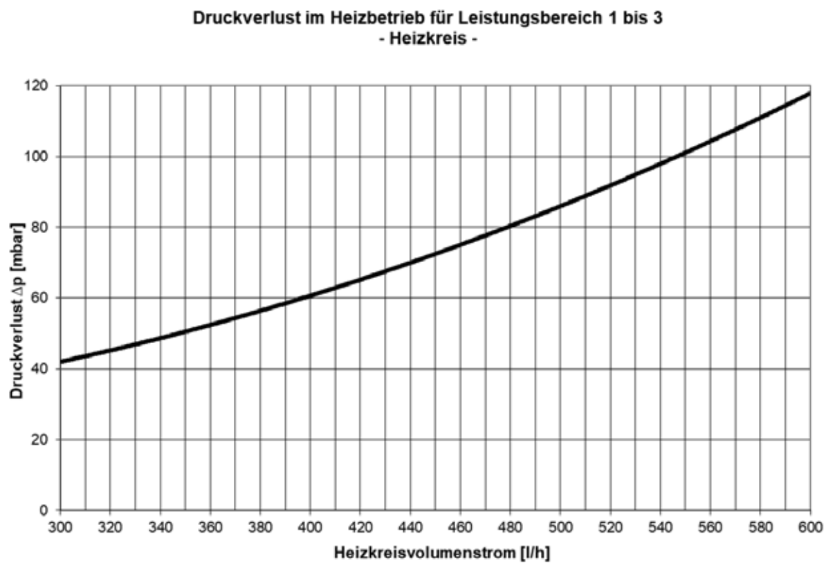
Abb. 30: Druckverlust im Heizbetrieb
