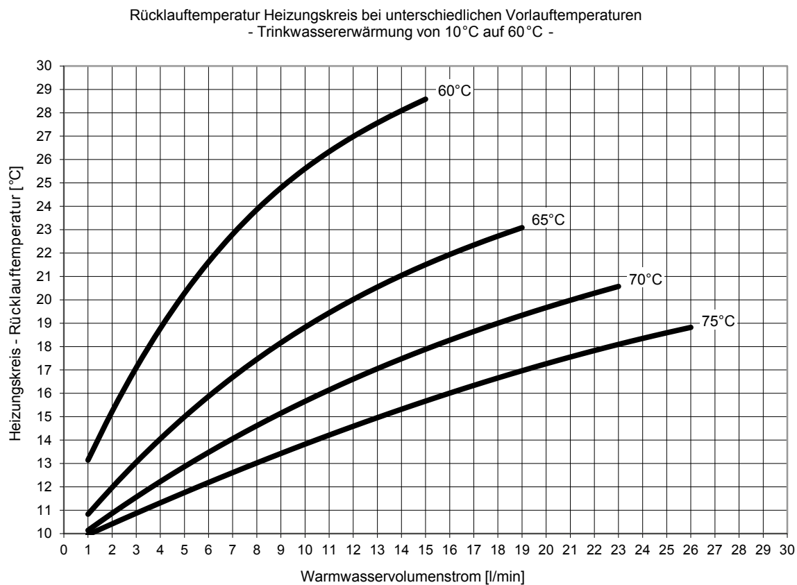
Abb. 47: Leistungsbereich 2, Trinkwassererwärmung auf 60 °C
