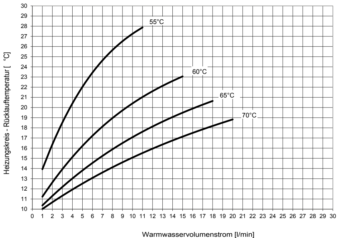
Rücklauftemperatur Heizungskreis bei unterschiedlichen Vorlauftemperaturen - Trinkwassererwärmung von 10 °C auf 55
