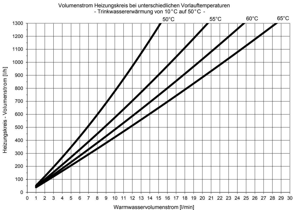
Abb. 42: Leistungsbereich 2, Trinkwassererwärmung auf 50 °C
