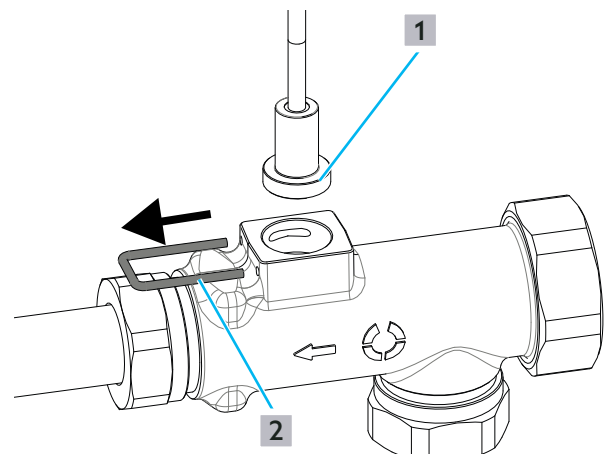
Abb. 23: Sicherungsklammer lösen
