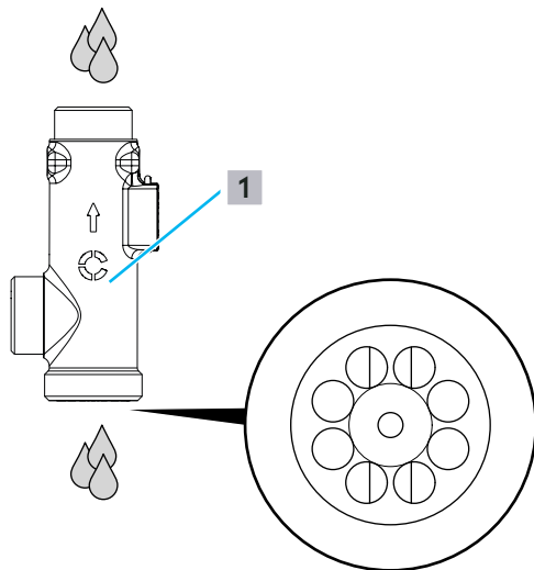
Abb. 25: Volumenstromsensor unter fließendem Wasser reinigen
