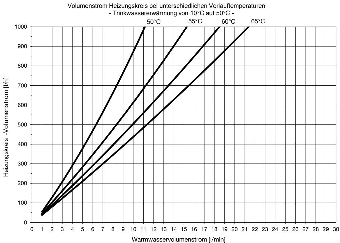
Abb. 35: Leistungsbereich 1, Trinkwassererwärmung auf 50 °C
