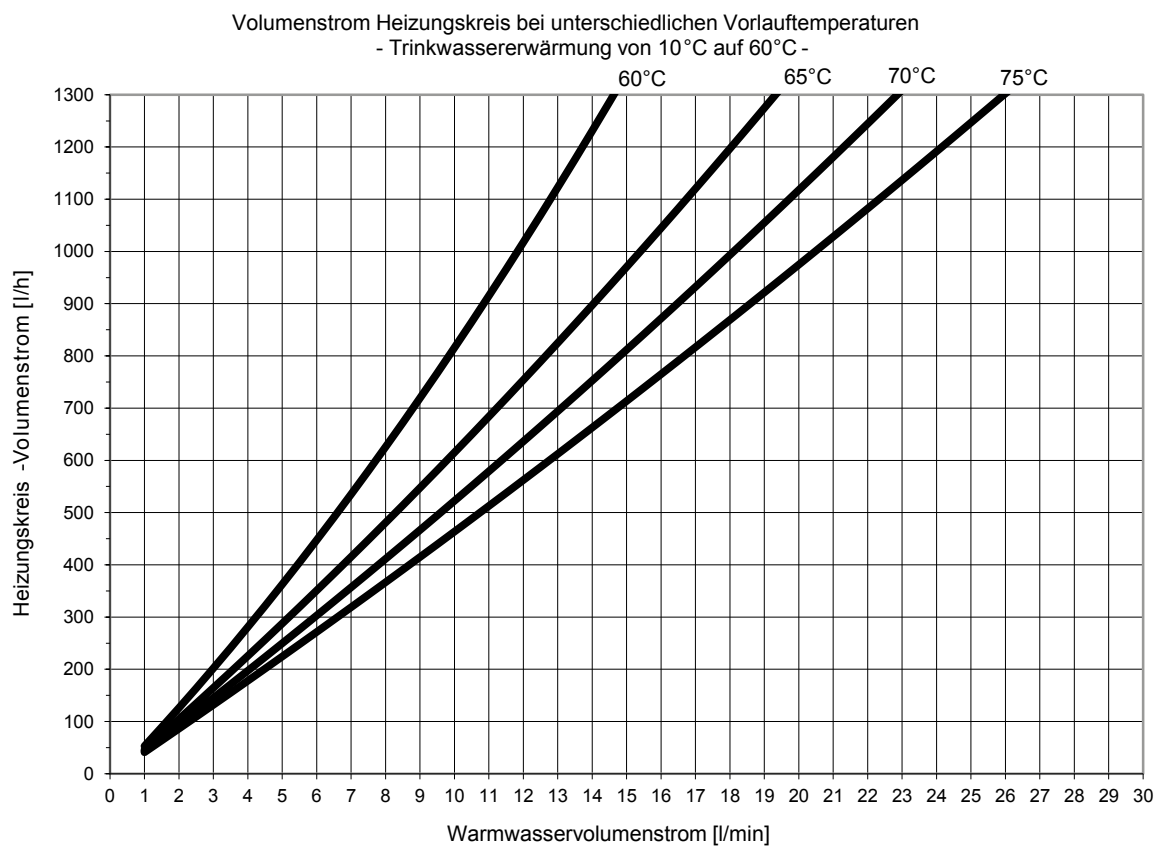
Abb. 46: Leistungsbereich 2, Trinkwassererwärmung auf 60 °C
