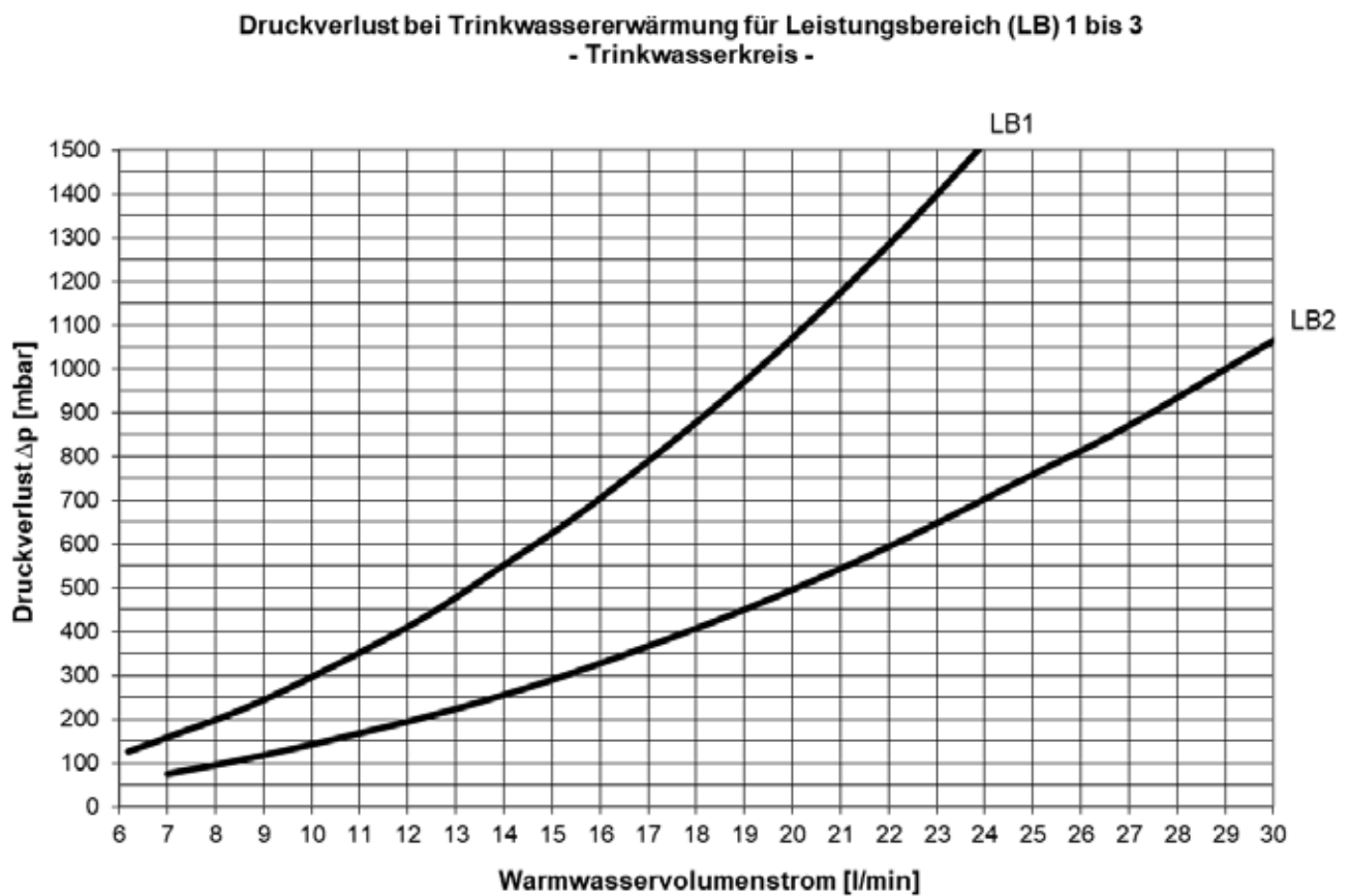
Abb. 31: Druckverlust im Trinkwasserkreis
