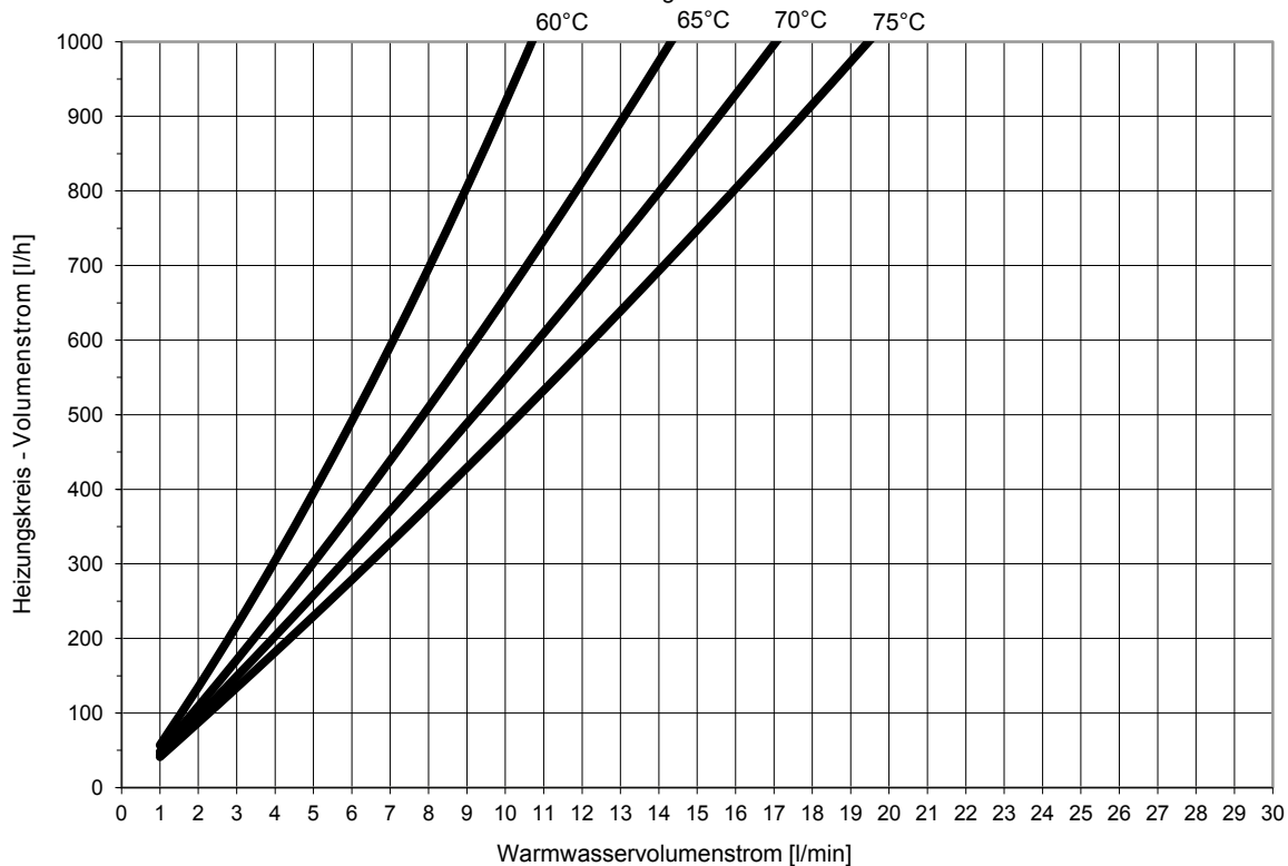
Abb. 38: Leistungsbereich 1, Trinkwassererwärmung auf 60 °C
