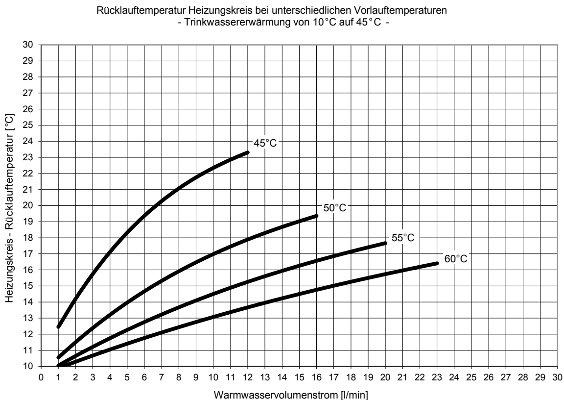
Abb. 34: Leistungsbereich 1, Trinkwassererwärmung auf 45 °C
