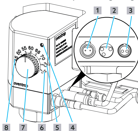
Abb. 4: Stellantrieb mit integrierter Trinkwassertemperaturregelung
