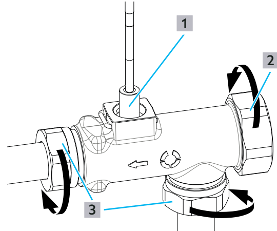
Abb. 26: Volumenstromsensor einbauen
