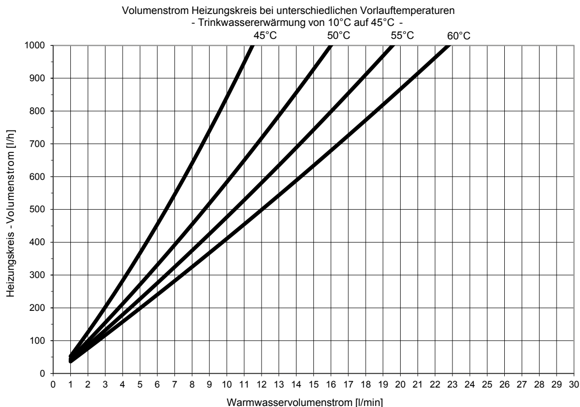
Abb. 33: Leistungsbereich 1, Trinkwassererwärmung auf 45 °C
