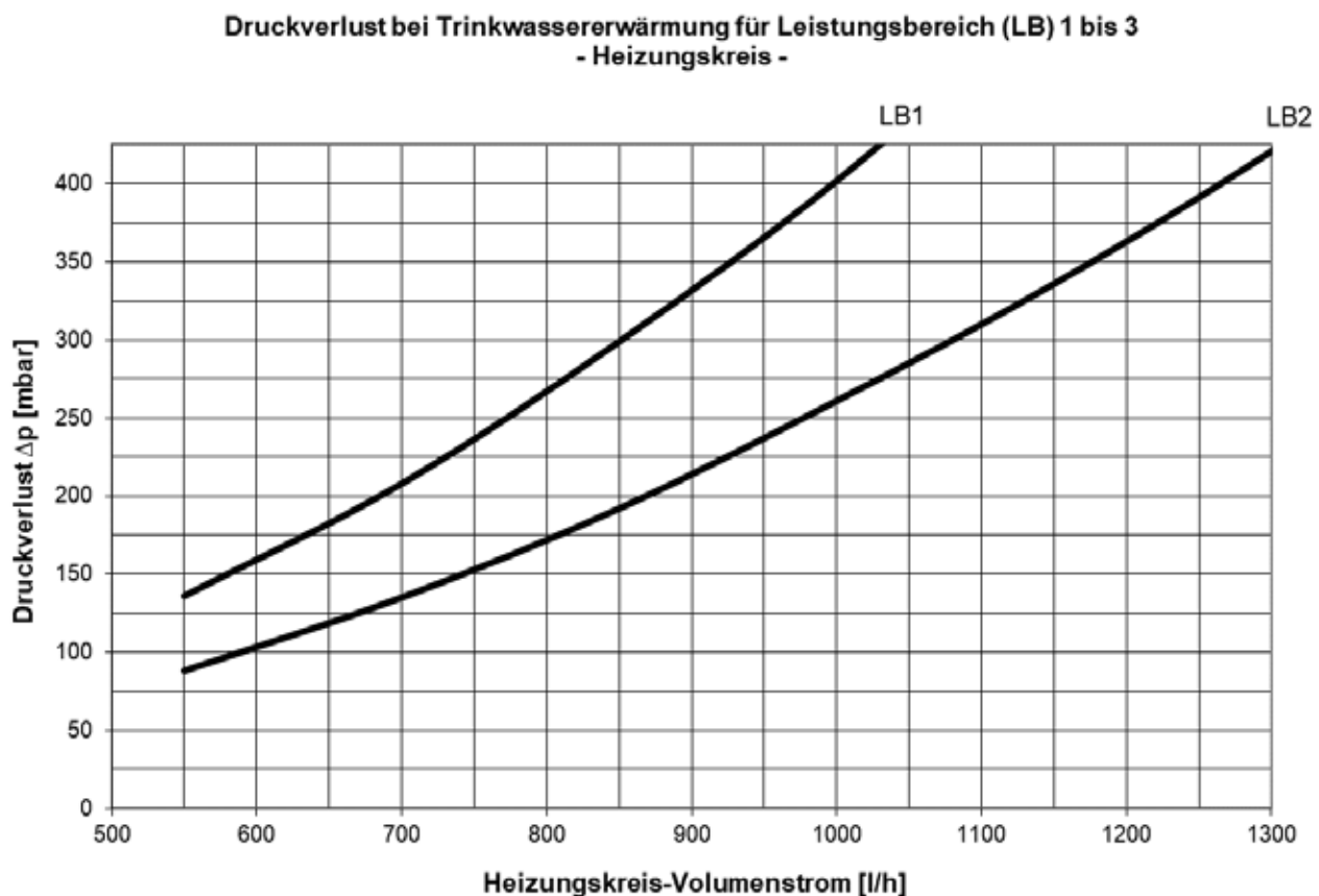
Abb. 32: Druckverlust im Heizungskreis
