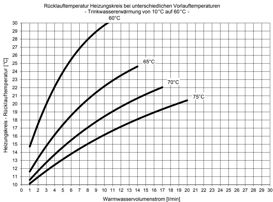
Abb. 39: Leistungsbereich 1, Trinkwassererwärmung auf 60 °C
