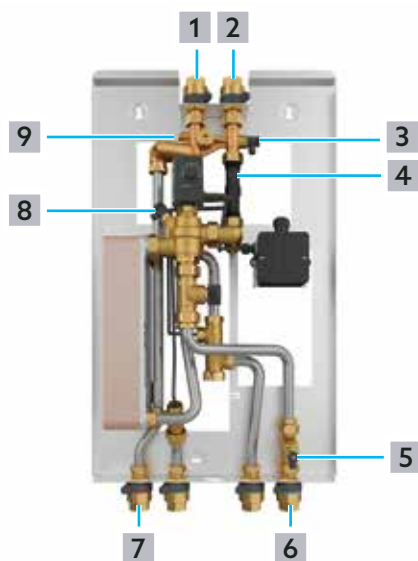
Abb. 11: Wärmezähler montieren
