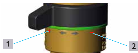
Abb. 17: Griffstellung geöffnet / geschlossen
