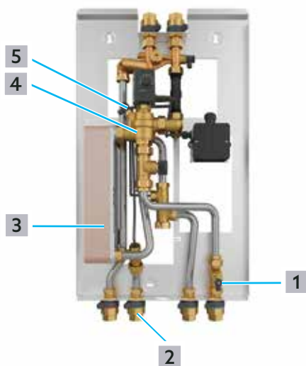
Abb. 21: Wärmeübertrager ausbauen und reinigen
