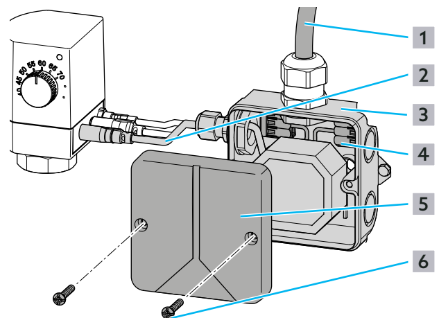
Abb. 13: Station elektrisch anschließen
