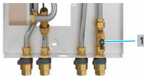
Abb. 28: Position Filtereinsatz Heizkreis-Rücklauf
