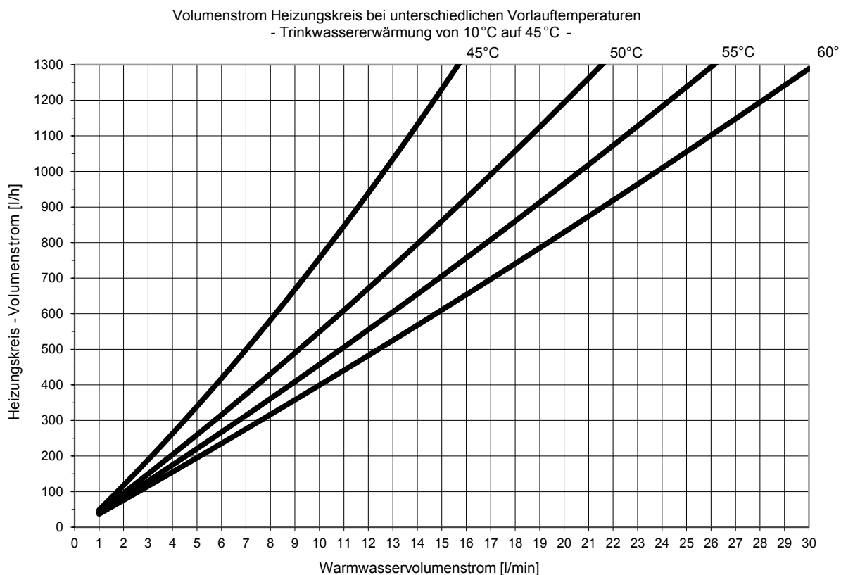
Abb. 40: Leistungsbereich 2, Trinkwassererwärmung auf 45 °C
