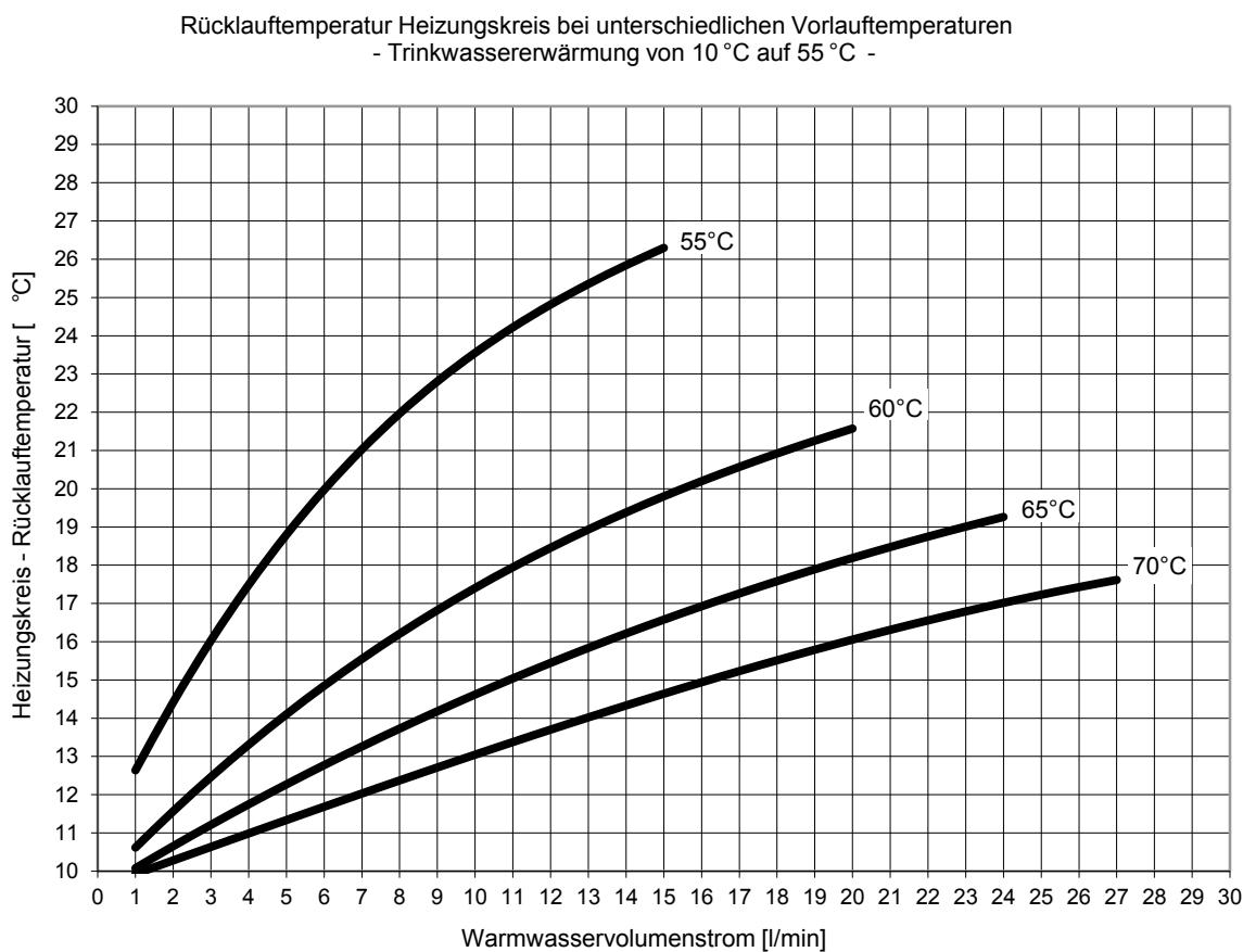
Abb. 45: Leistungsbereich 2, Trinkwassererwärmung auf 55 °C
