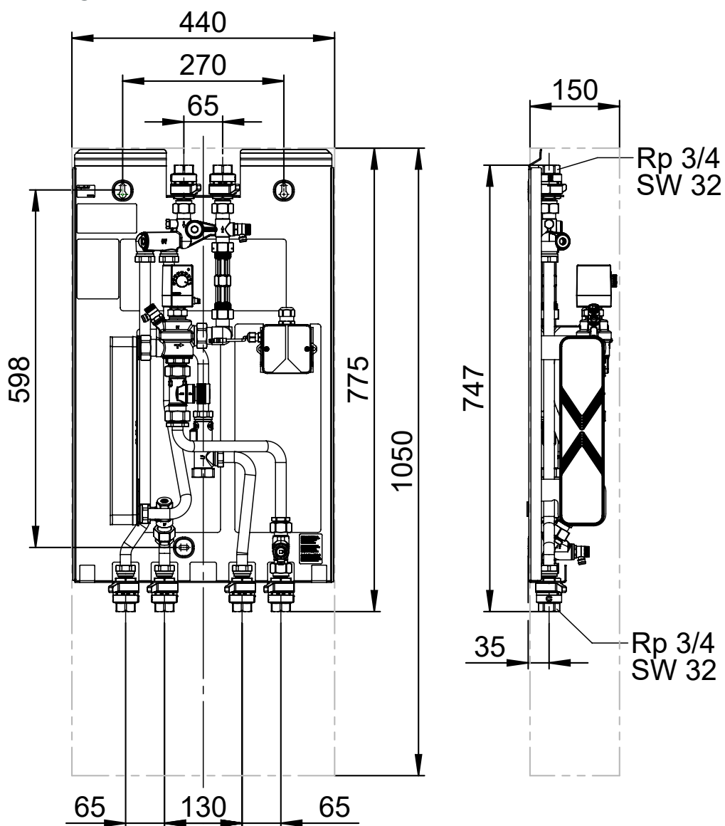
Abb. 5: Abmessungen
