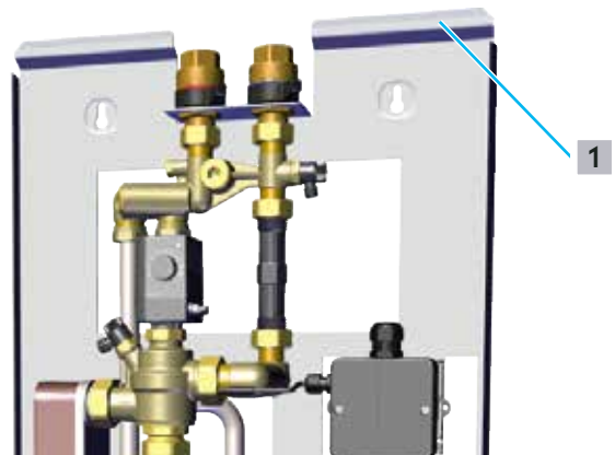
Abb. 19: Aufputzhaube montieren
