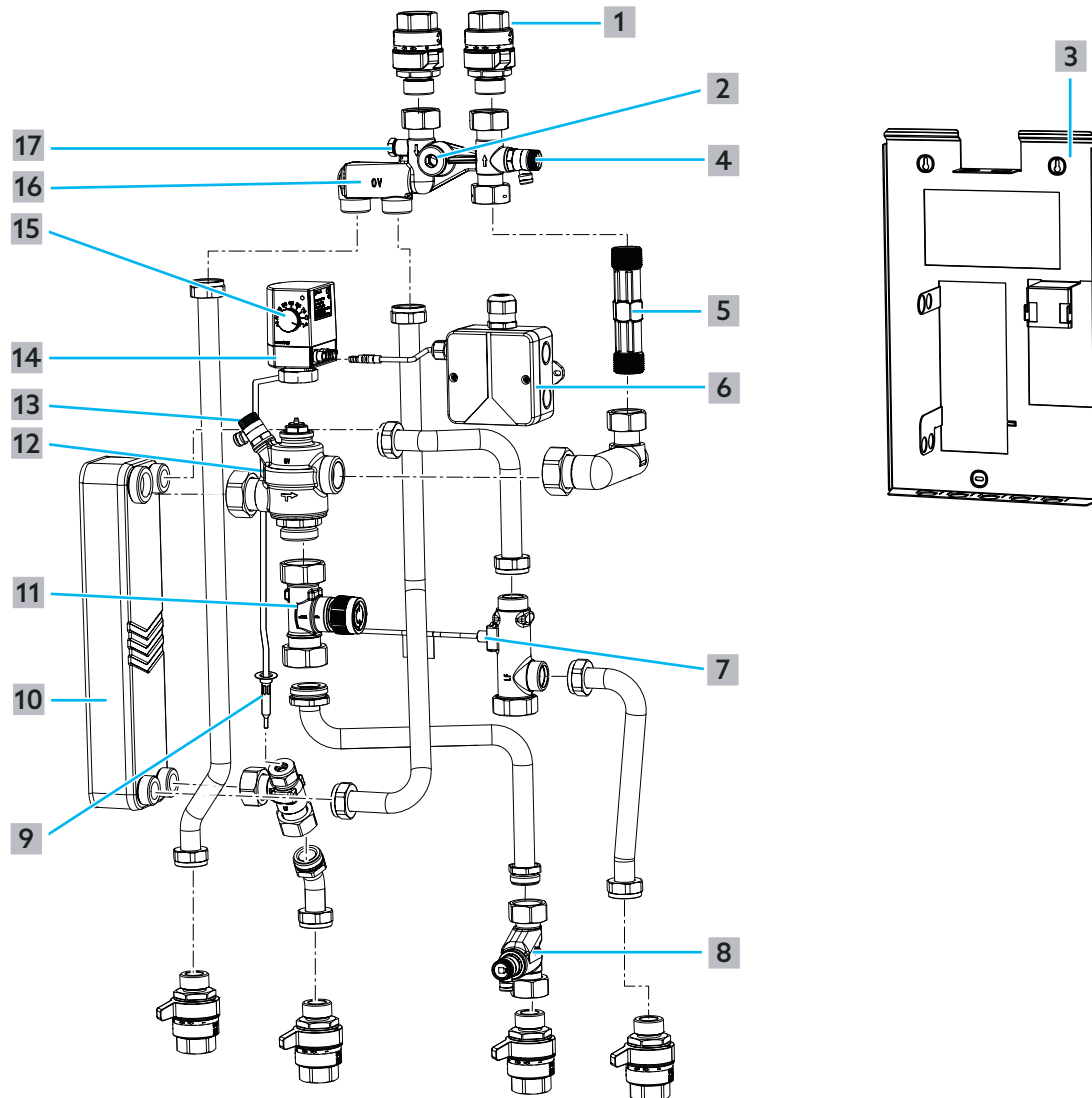
Abb. 3: Übersicht Station Regudis W-HTE GT
