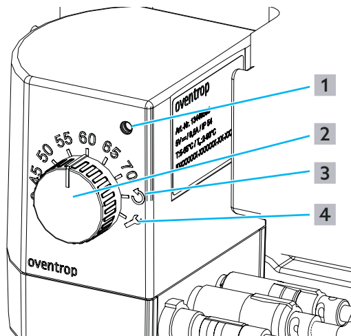
Abb. 20: Statusmeldungen und Fehlermeldungen am Stellantrieb
