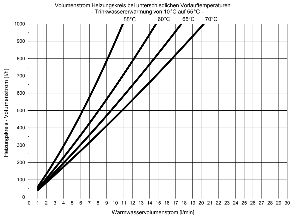
Abb. 36: Leistungsbereich 1, Trinkwassererwärmung auf 55 °C
