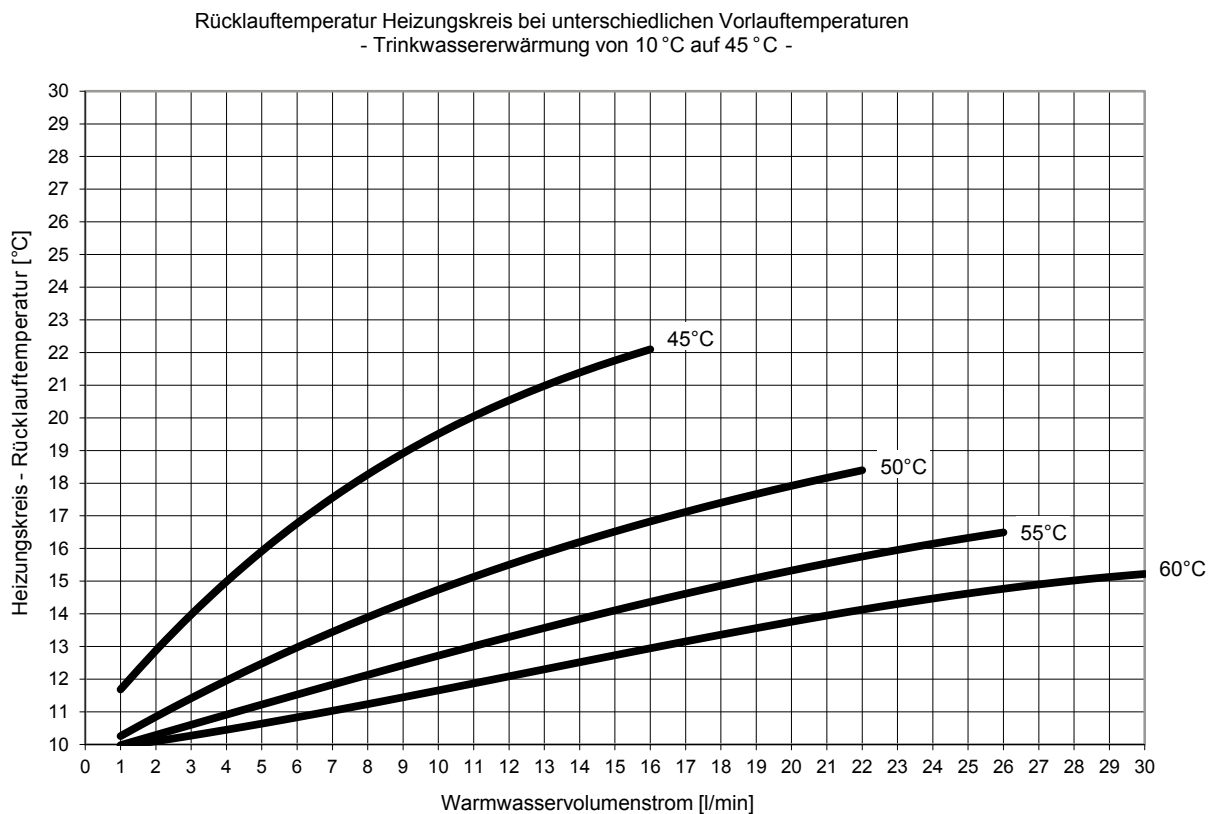
Abb. 41: Leistungsbereich 2, Trinkwassererwärmung auf 45 °C
