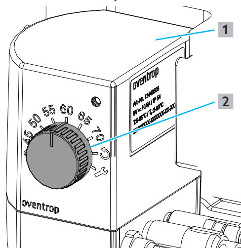
Abb. 29: Warmwassertemperatur einstellen
