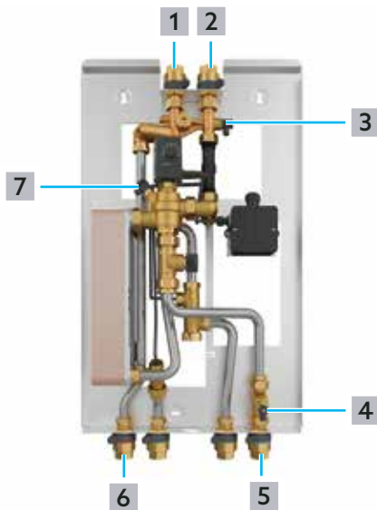
Abb. 14: Heizkreis füllen und entlüften
