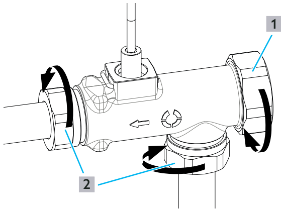
Abb. 24: Volumenstromsensor ausbauen
