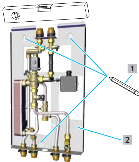
Abb. 9: Station ausrichten und anzeichnen
