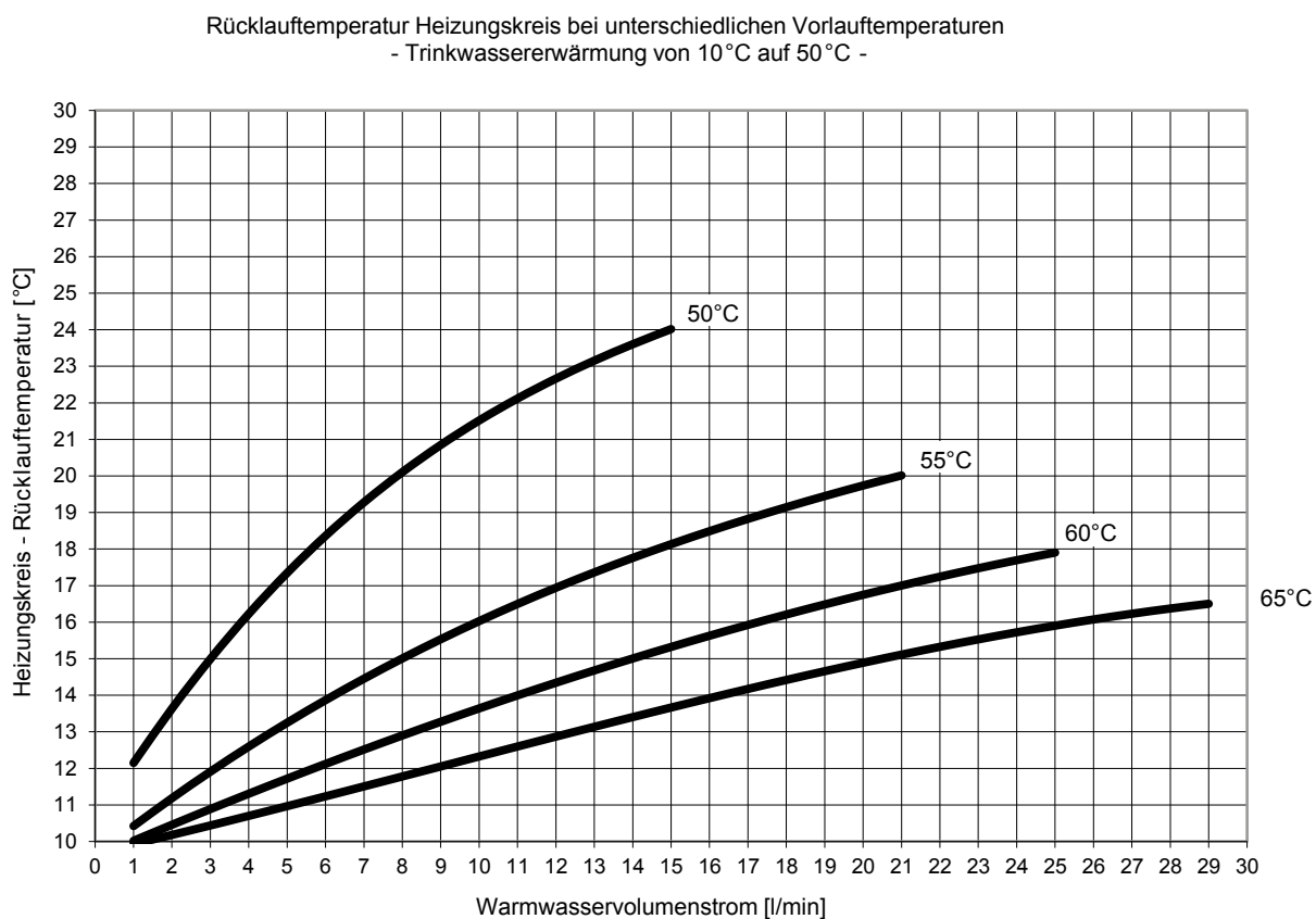
Abb. 43: Leistungsbereich 2, Trinkwassererwärmung auf 50 °C
