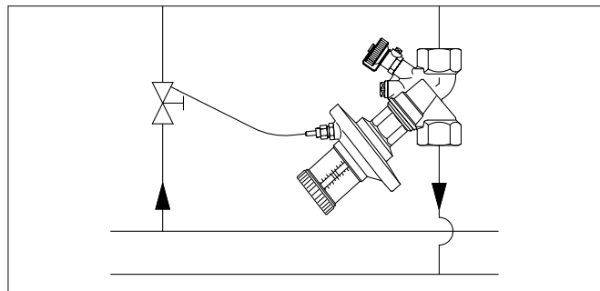
Příklad: Regulace diferenčního tlaku v zařízeních s přednastavitelnými termostatickými ventily (smyčky se středním až větším průtokem)
