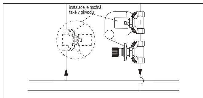
Příklad: Regulace průtoku pomocí kombinace armatur, regulátoru diferenčního tlaku „Hycocon DP“ a smyčkového ventilu „Hycocon TM“
