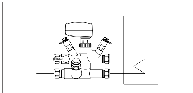
Příklad: Regulace zařízení jen s jedním čtyřcestným regulačním ventilem „Cocon 4“.
