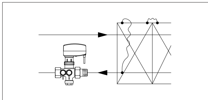
Příklad: Zařízení stropní chladicí soustavy pro snížení prostorové teploty
