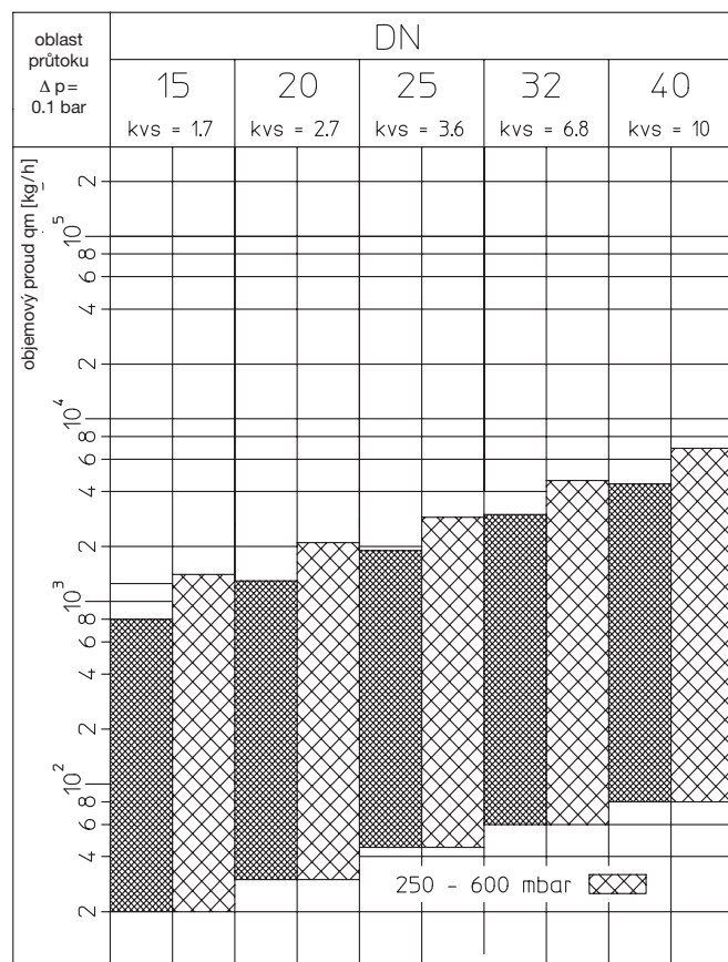
„Hycococon DP“ (50–300 mbar) „Hycococon DP“ (250–600 mbar)
