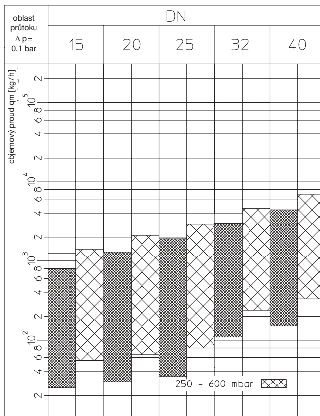
„Hycococon DP“ (50–300 mbar)/„Hycococon V“ „Hycococon DP“ (250–600 mbar)/„Hycococon V“
