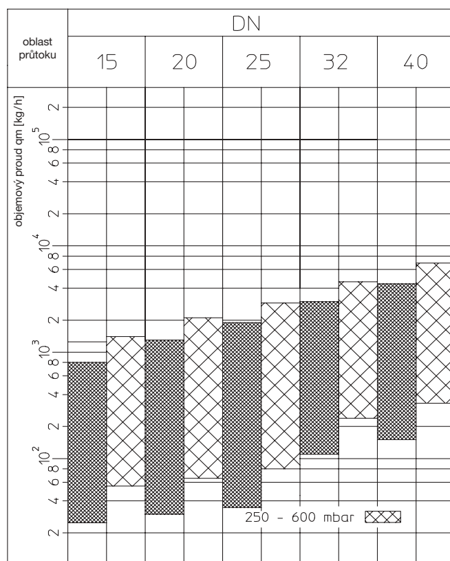
„Hycocon DP“/„Hycocon TM“ se servopohonem
