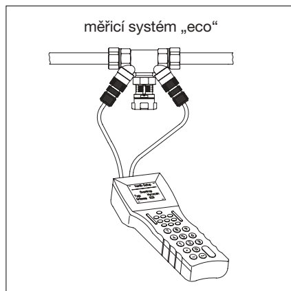
Nastavení na smyčkovém regulačním ventilu „Hycoco V“.
