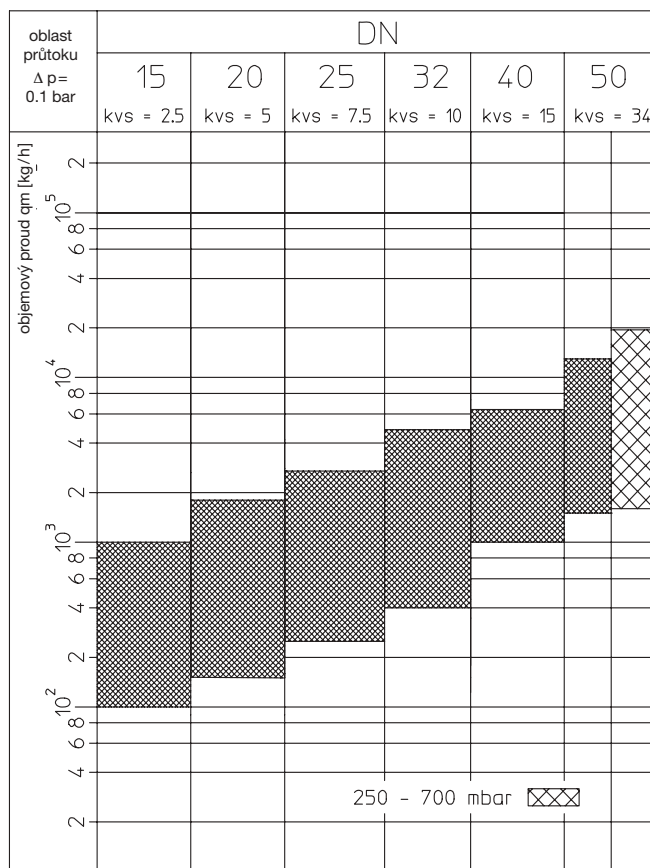
„Hydromat DP“ (50–300 mbar) „Hydromat DP“ (250–700 mbar)
