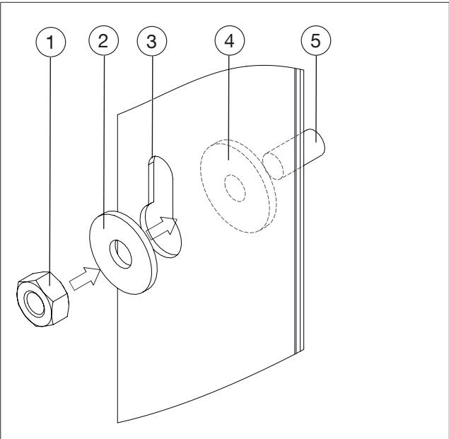
Fig. 6: Points de fixation de la station d'appartement Regudis W-HTF
