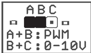
Jumperstellung für PWM-Signal
