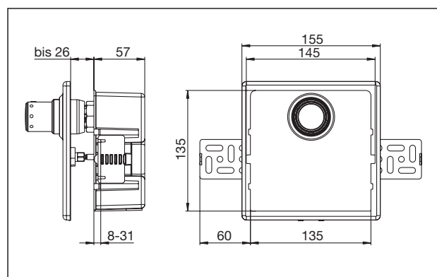
Maße „Unibox TSH“, Bautiefe 57 mm
