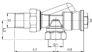
Winkelackergehäuse
