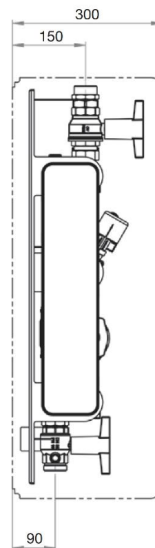
Abmessungen Regumaq X-70 (Seite)
