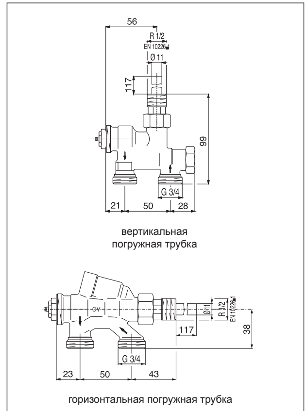
Вентили с погружной трубкой (для одноконтурных/двухконтурных систем)
