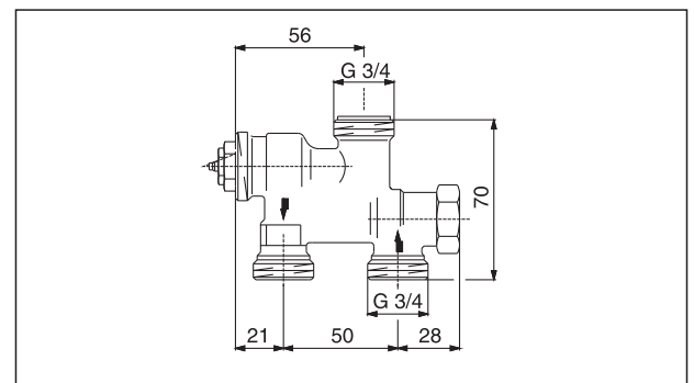
Вентиль „TKM“ (для одноконтурных/двухконтурных систем)
