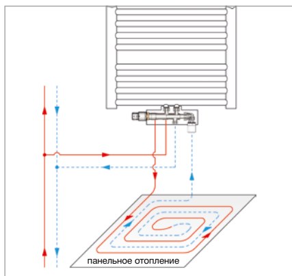
Пример установки „Multiblock T-RTL“ с панельным отоплением
