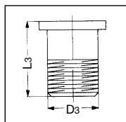
Schroefdraadtules
