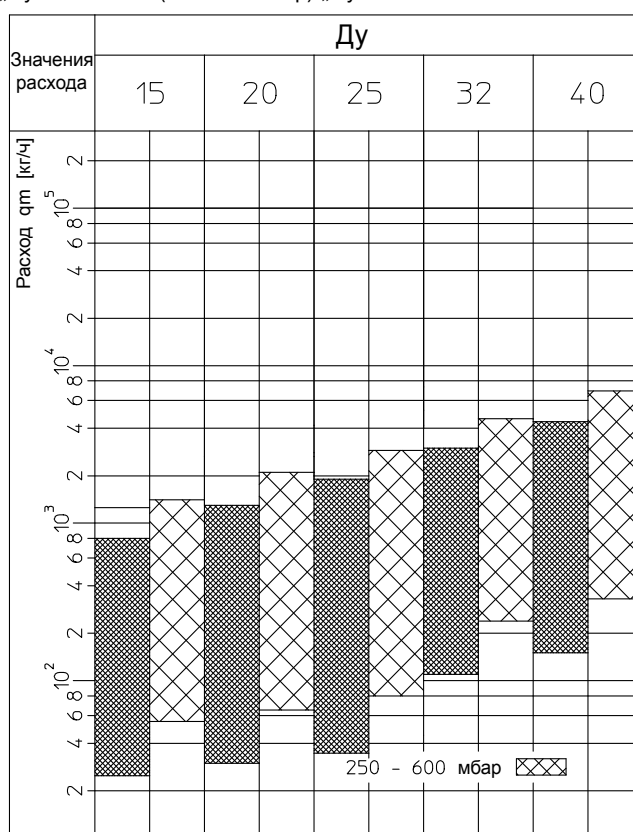
„Нусосокоп DTZ“ (50–300 мбар)/„Нусосокоп VTZ“ „Нусосокоп DTZ“ (250–600 мбар)/„Нусосокоп VTZ“
