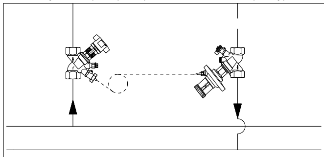
Пример: Регулирование перепада давления с ограничением расхода в системе без преднастраиваемых термостатических вентилей.
