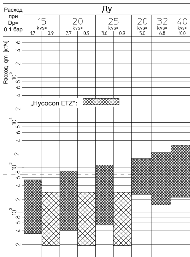
„Hycococon ATZ/VTZ/ETZ/HTZ“
