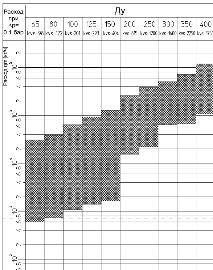
„Hydrocontrol VFC/VFR/VFN/VGC“
