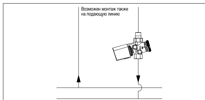
Пример: Регулирование расхода с помощью вентиля „Cocon QTZ“.
