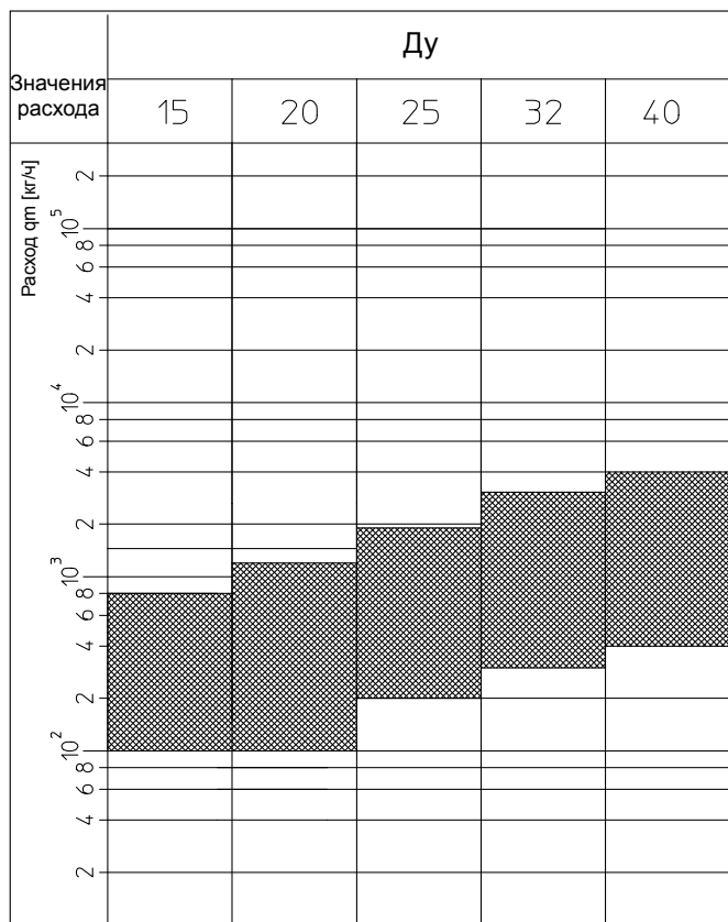
„Hydromat QTR“
