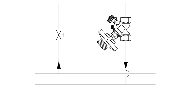
Пример: Регулирование расхода напр., в системе охлаждения. Преднастройка на регуляторе легко считывается.
