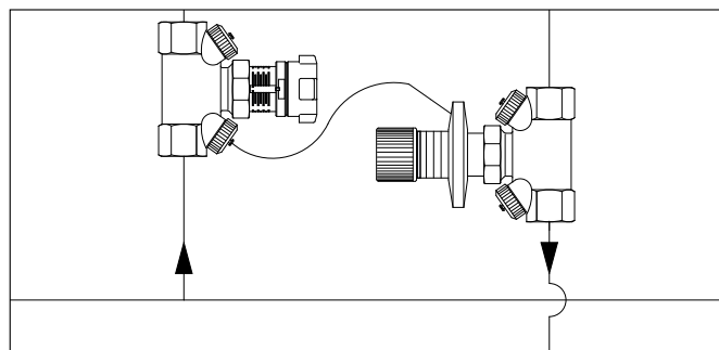
Пример: Регулирование перепада давления и ограничение расхода в системе без преднастраиваемых термостатических вентилей.
