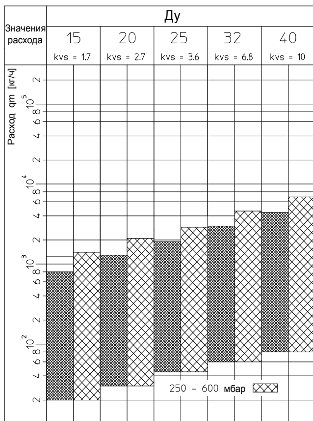
„Нуссоп DTZ“ (50–300 мбар) „Нуссоп DTZ“ (250–600 мбар)
