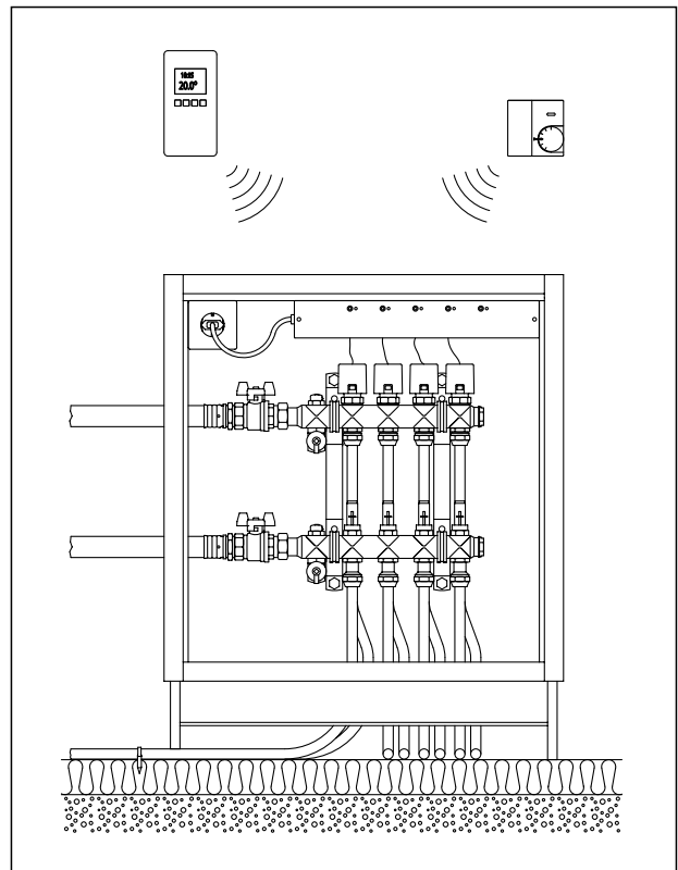
Przykład instalacji
