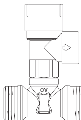
Fig. 7: Soupape de sécurité 6 bars, réf. OV 136 41 40
