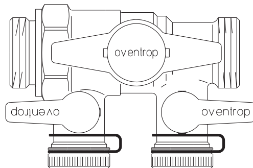
Bild 6: Befüll- und Spülmaterie, OV-Art.-Nr. 136 30 51
