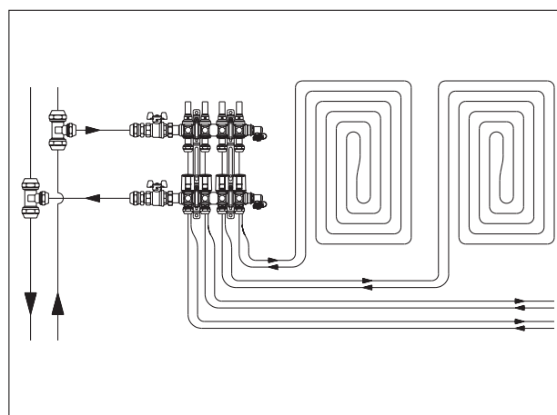
System-Darstellung „Multidis“ Edelstahl-Verteiler
