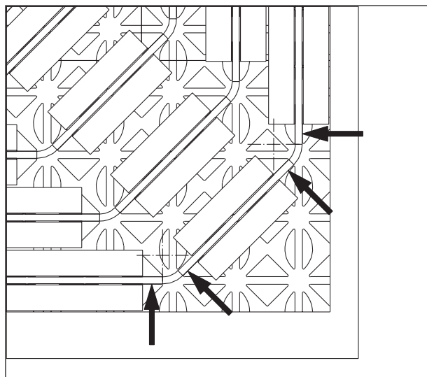
90°-Bogen bei schneckenförmiger Verlegung
