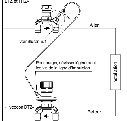
Illustr. 6.2: «Hycoco DTZ» Montage sur le retour
