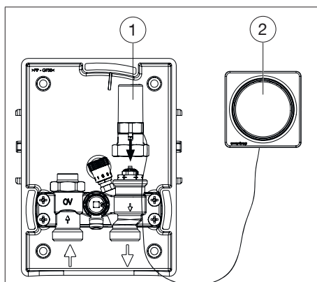
Fig. 8: Montage de la tête thermostatique avec commande à distance
