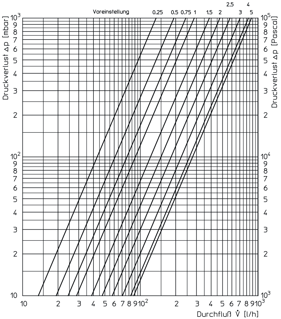
Abb. 12: Diagramm Reguliereinsatz, 2K P-Abweichung, Bypass Voreinstellung 2,3 (75%)
