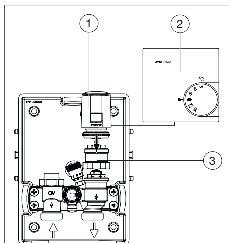
Fig. 9: Montage du thermostat d'ambiance avec moteur
