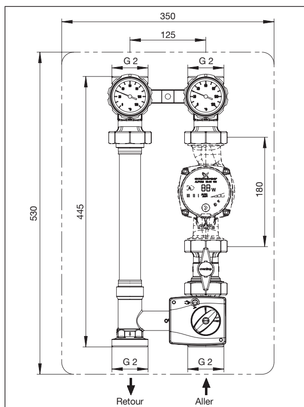
Encombres Regumat M3-180 DN 32
