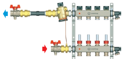
Abb. 6: Montagebeispiel Wärmemesszähler-Anschluss-Set, Durchgangsform
