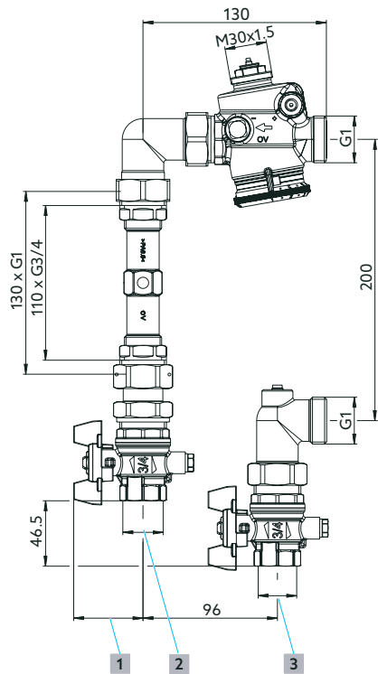
Abb. 3: Abmessungen Eckausführung
