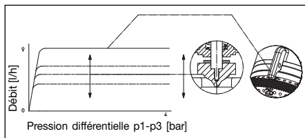
Fig. 5.6 Ligne caractéristique du débit pour pré-régulages différents
