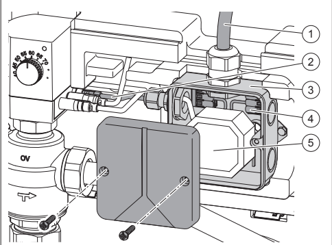
Abb. 1: Aufbau
