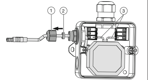
Abb. 2: Aufbau Zugentlastung
