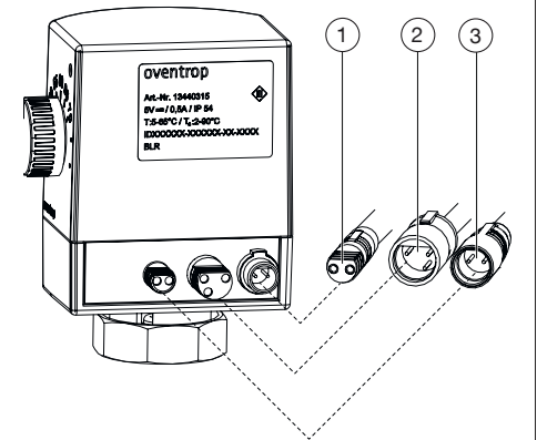
Abb. 3: Steckverbindungen
