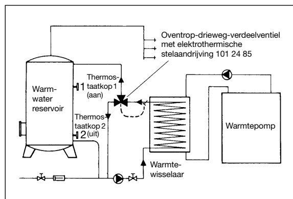
Schematische doorsnede
