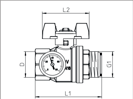
Abb. 5: Maße Kugelhahn
