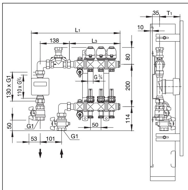
Fig. 2: Set di collegamento contacalorie, versione dritto, fornitura e montaggio dei componenti su lato dx.
