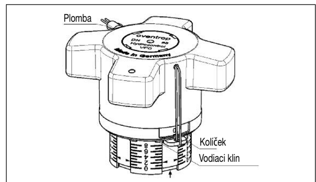
Obr. 7.2 Blokovanie ručného koleska
