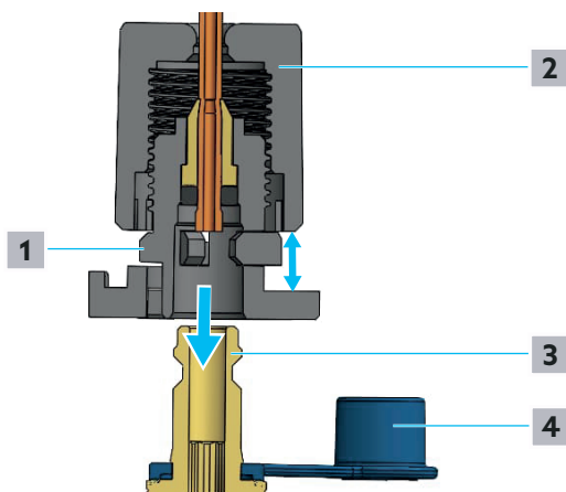
Bild 6: Anslutning av impulsledningen till partnerventilen
