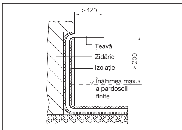
Secțiune, racordarea circuitului de încălzire
